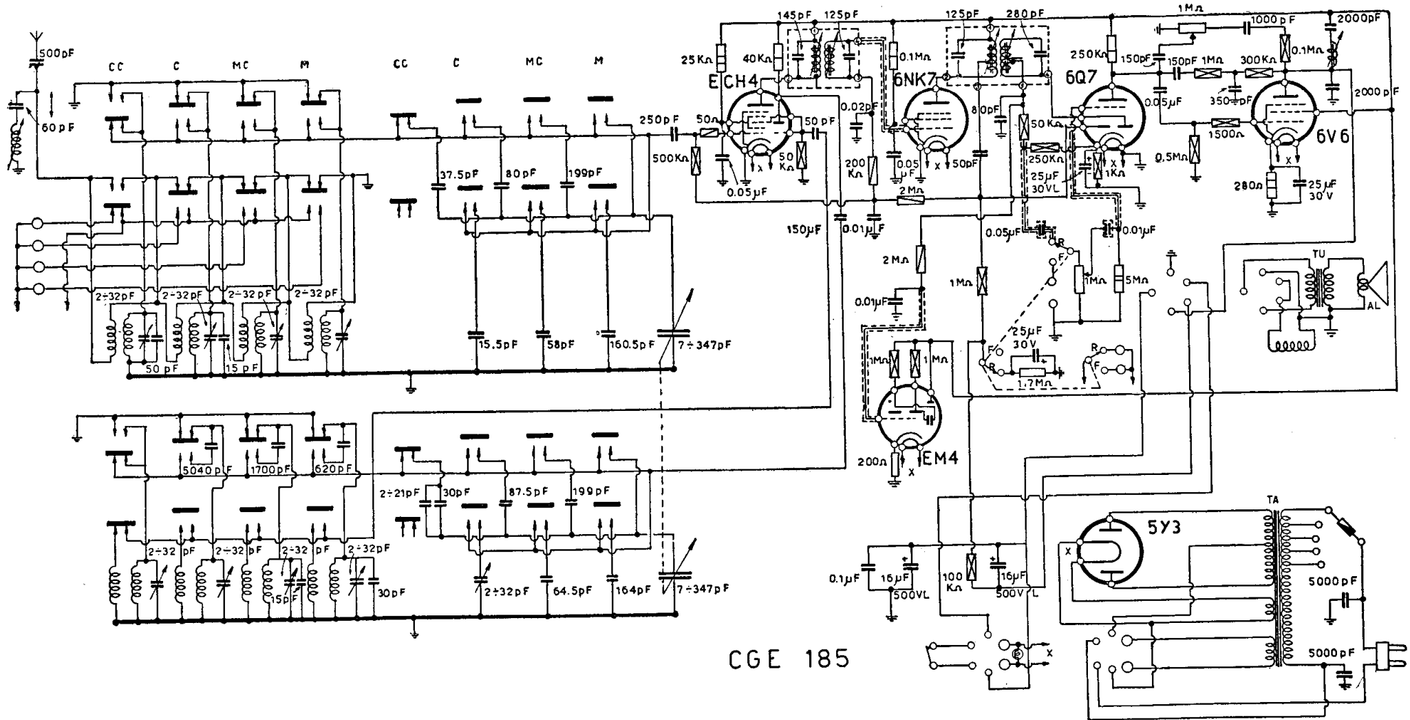
COMPAGNIA GENERALE DI ELETTRICITÀ - Mod. 185 - Due gamme onde medie e due gamme onde corte. Nello schema è inserita la gamma cortissime (CC). Media frequenza 468 kc. Potenza d'uscita 4 W.
